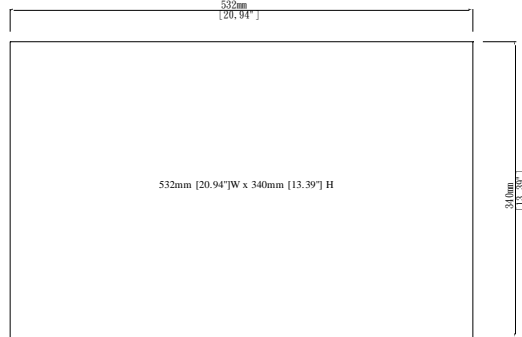
Cutout Dimensions
