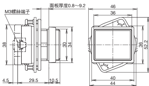
螺絲端子：M3
