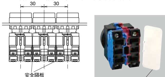
安全隔板 接點塊之間務必使用 1 個安全隔板 (HW-VU1 型)
