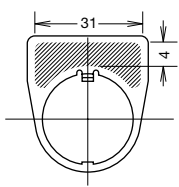
①標準型 (NSA / NFSO 型)
