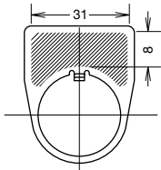
②大蘑菇頭形 (NSALO 型)
