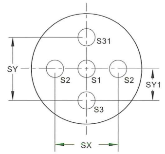
底面(安裝面)BOTTOM
